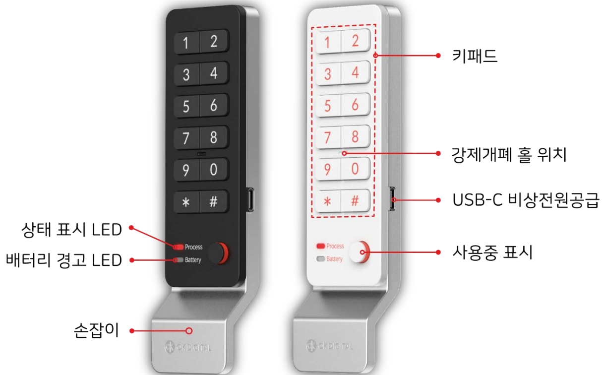
전면부(프론트)
